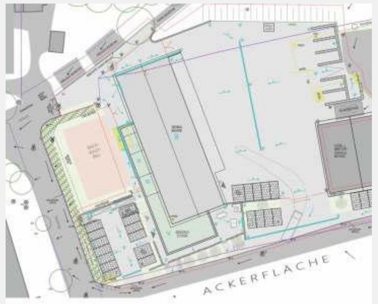
Lageplan mit neuem Bauhof
